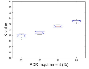
Fig. 14. The value of the parameter K
